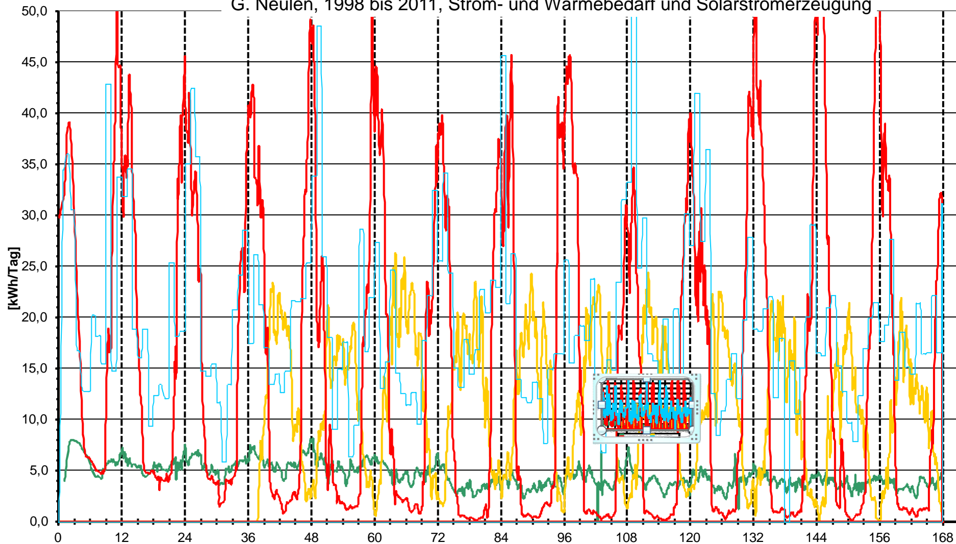
G. Neulen, 1998 bis 2011, Strom- und Wärmebedarf und Solarstromerzeugung
